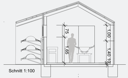
Querschnitt aus dem Bauplan zur neuen Werkstatt
